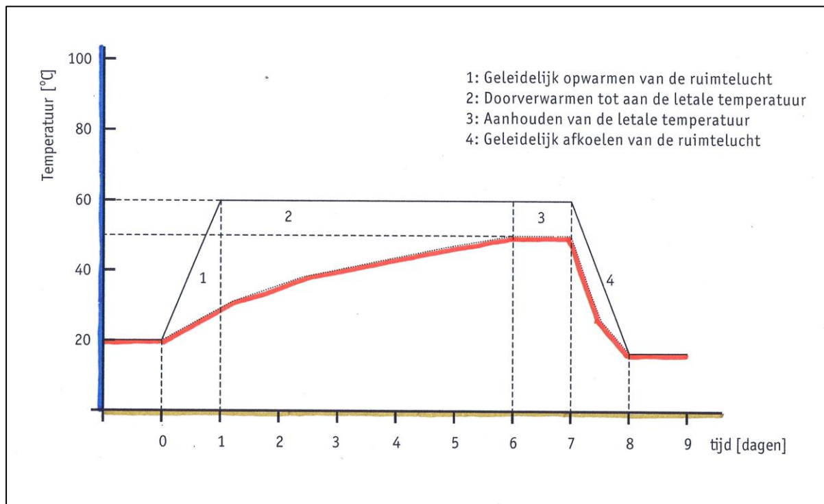
Afb 3 Grafiek tijdsduur als voorbeeld van een behandeling met hete lucht
