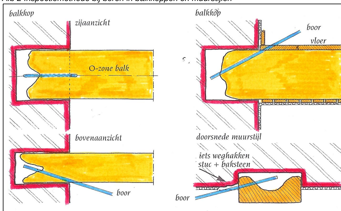
Afb 2 Inspectiemethode bij boren in balkkoppen en muurstijlen
