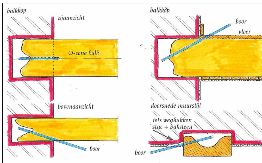
Figuur 1 Inspectiemethode bij boren in balkkoppen en muurstijlen
