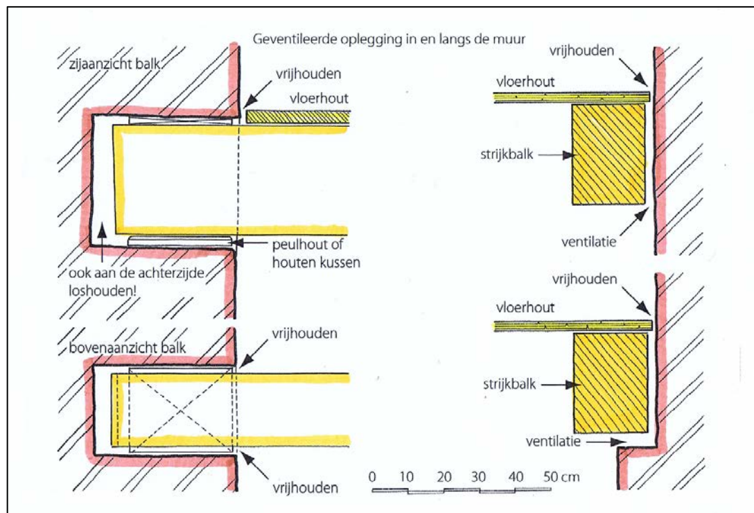
Figuur 3 Geventileerde oplegging van balkkoppen en strijkbeuken
