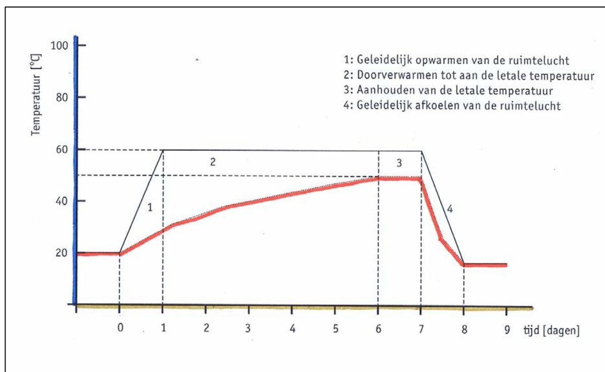
Figuur 2 Grafiek tijdsduur als voorbeeld van een behandeling met hete lucht
