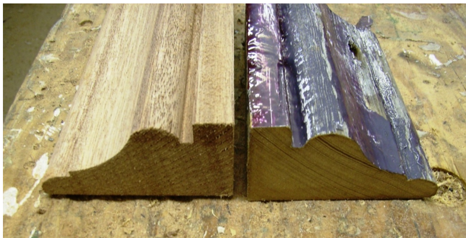
Gekopieerd lijstprofiel. Het origineel is niet ontverfd voor het kopiëren, wat afwijkingen kan veroorzaken in de maatvoering. Ook is een niet-geëigende houtsoort gebruikt (meranti).
